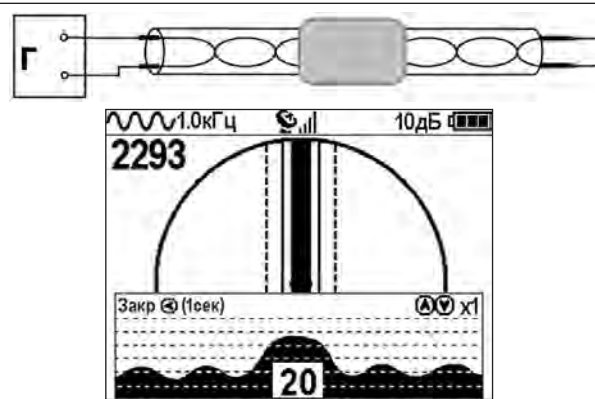
Рис.А.2 Муфта
