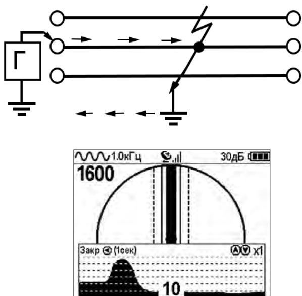
Рис.А.3 КЗ-однофазное
