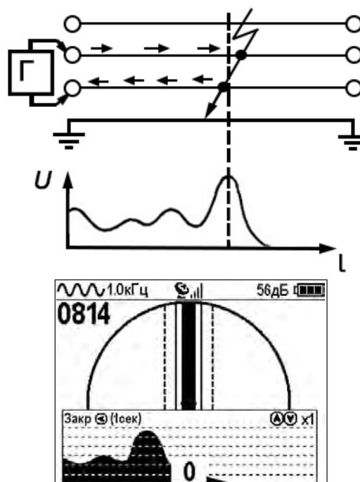
Рис.А.4 КЗ-двухфазное
